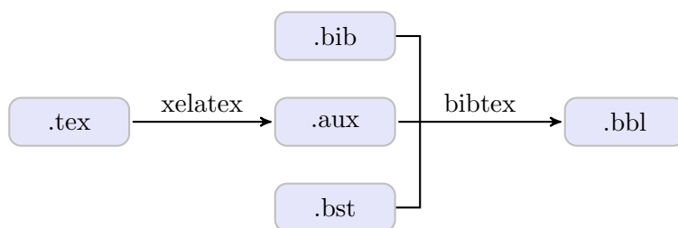
图 10.1: BibTeX 的编译
